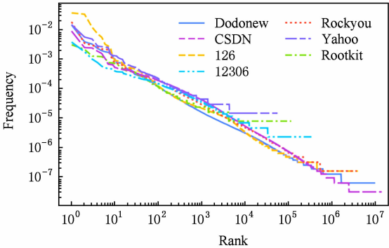
Fig. 1 Human-chosen passwords follow Zipf's law. 图 1 人类生成的口令服从 Zipf 分布
