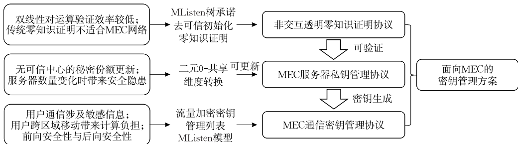
图 2 主要行文逻辑
