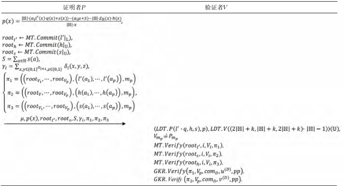
图 3 非交互零知识可验证多项式委托
